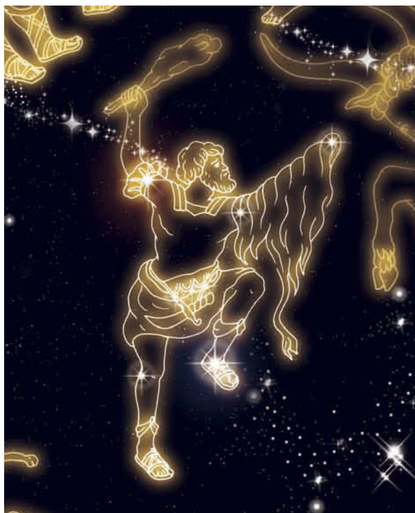
一等星2個、二等星5個を含む華やかなオリオン座。
