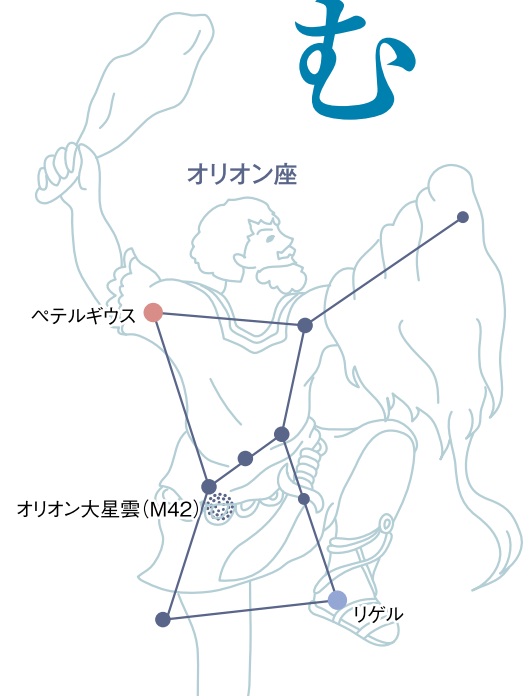
一等星2個、二等星5個を含む華やかなオリオン座。
