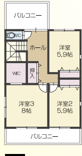
A棟 2F
