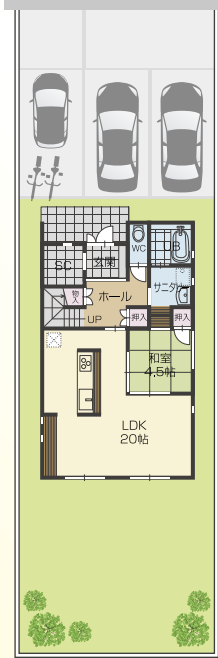
A棟 1F
